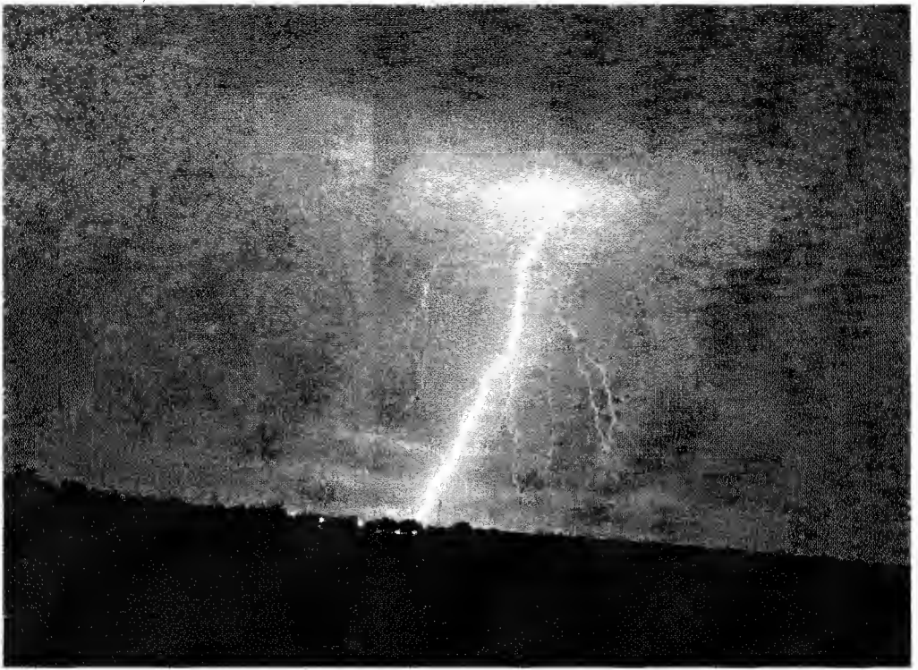
صورة للبرق الذي يحدث في نطيق المناخ (بين السماء والأرض)
